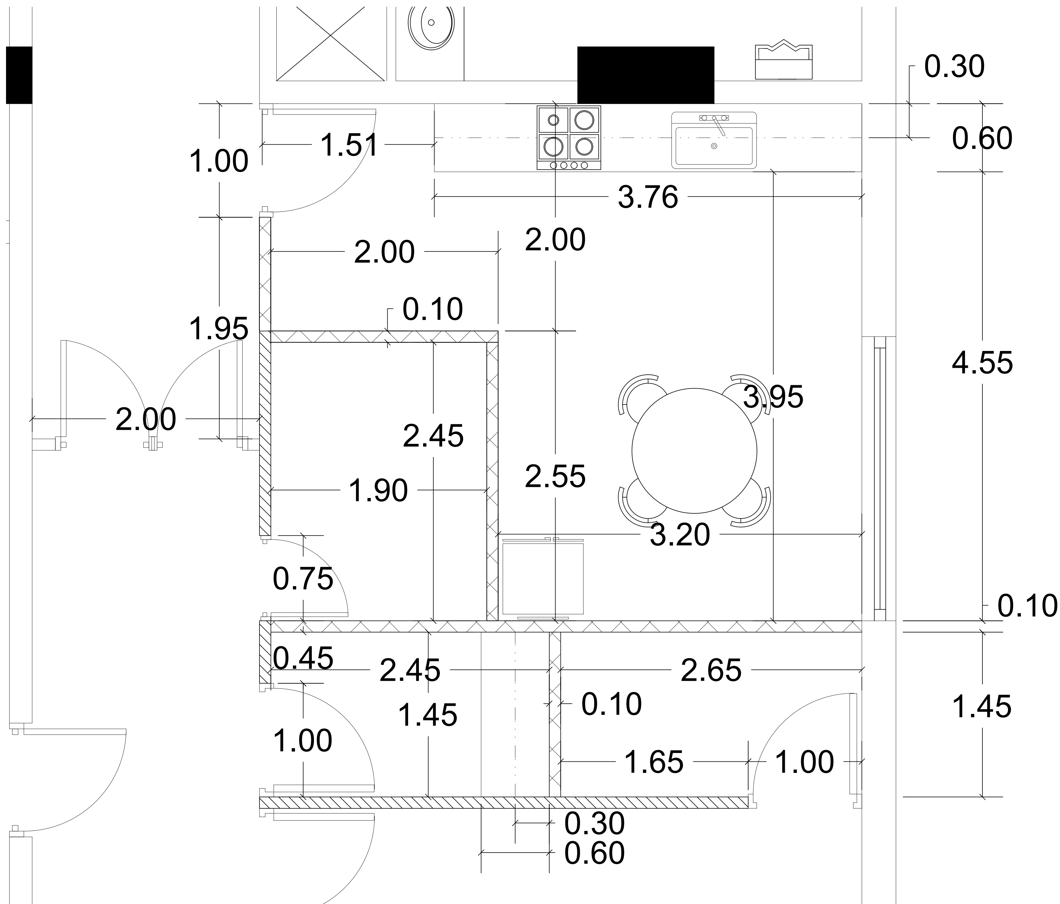
PLANTA PROPUESTA COCINA DIMENSIONADA 4
