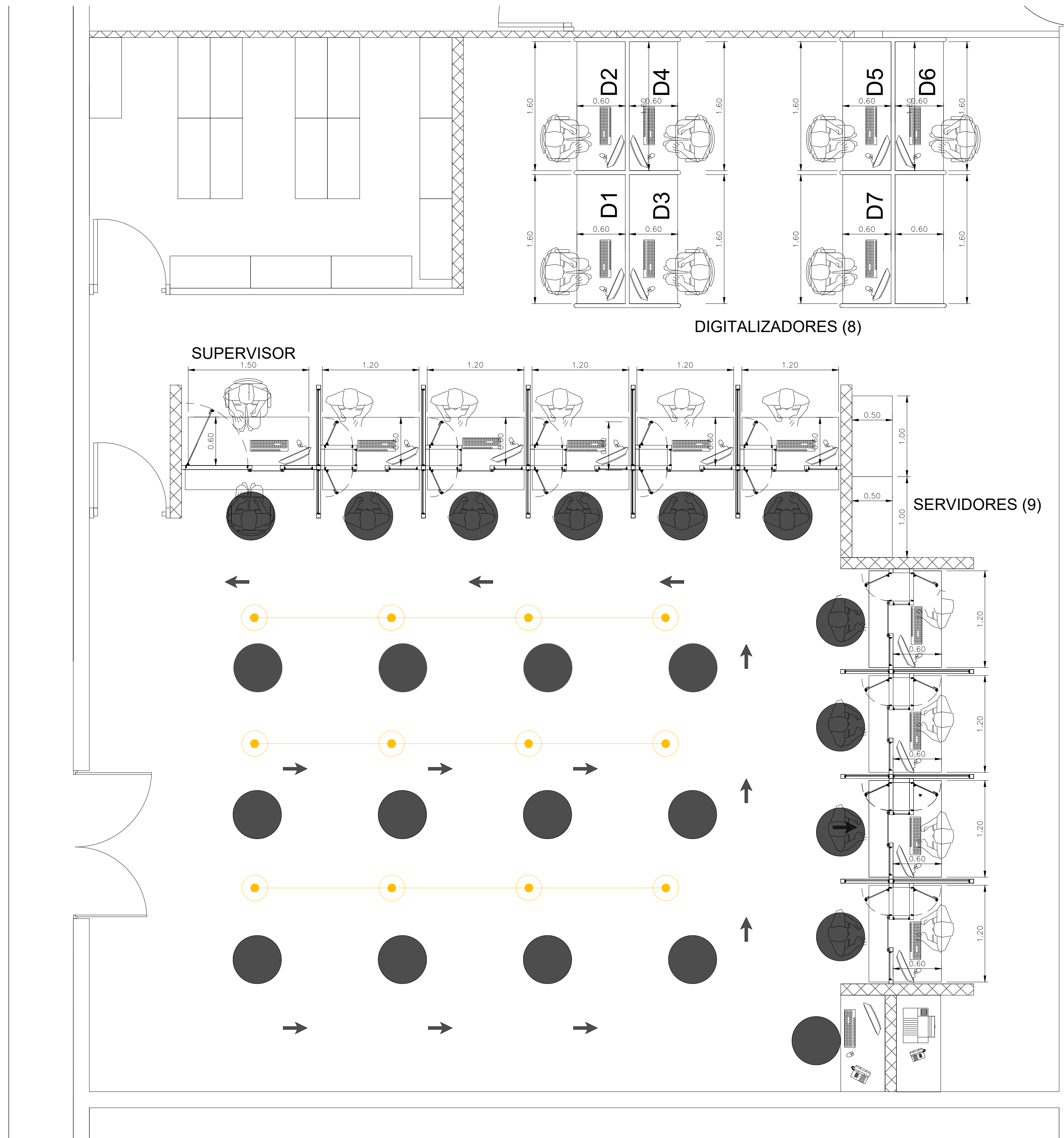
VISTA AMPLIADA PLANTA ARQUITECTONICA PROPUESTA RECEPCION DE DOCUMENTOS NIVEL 1
