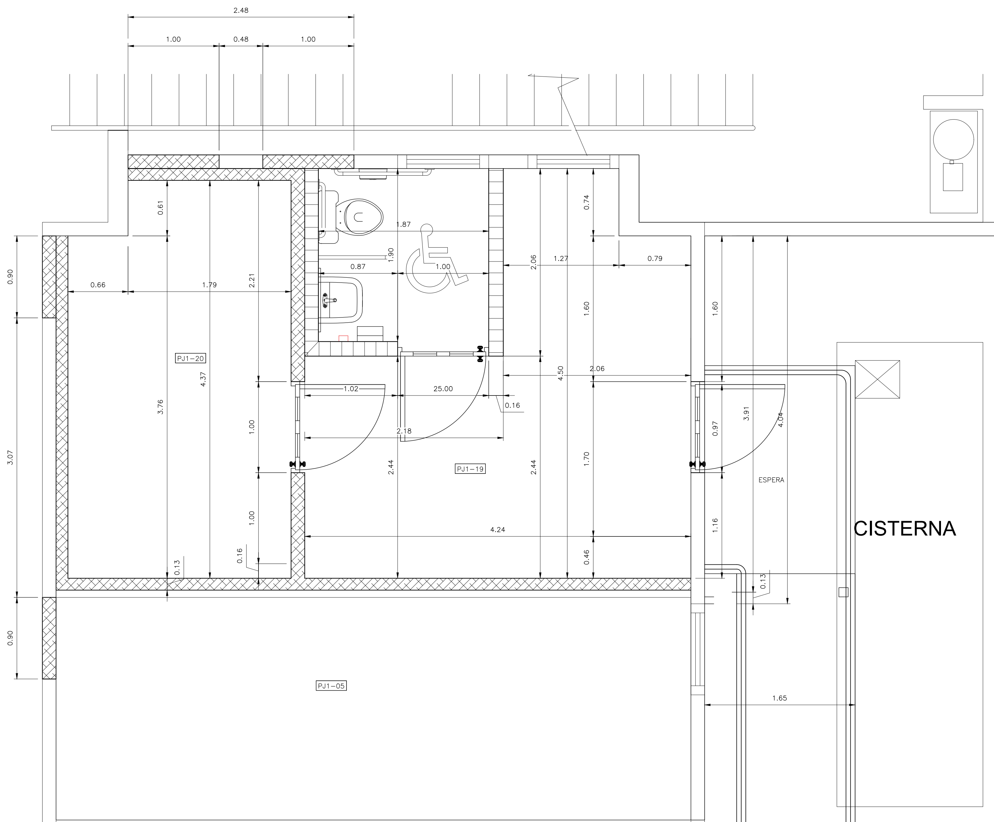
VISTA AMPLIADA PROPUESTA DIMENSIONADA SALA DE ENTREVISTAS ESCALA: 1:25
