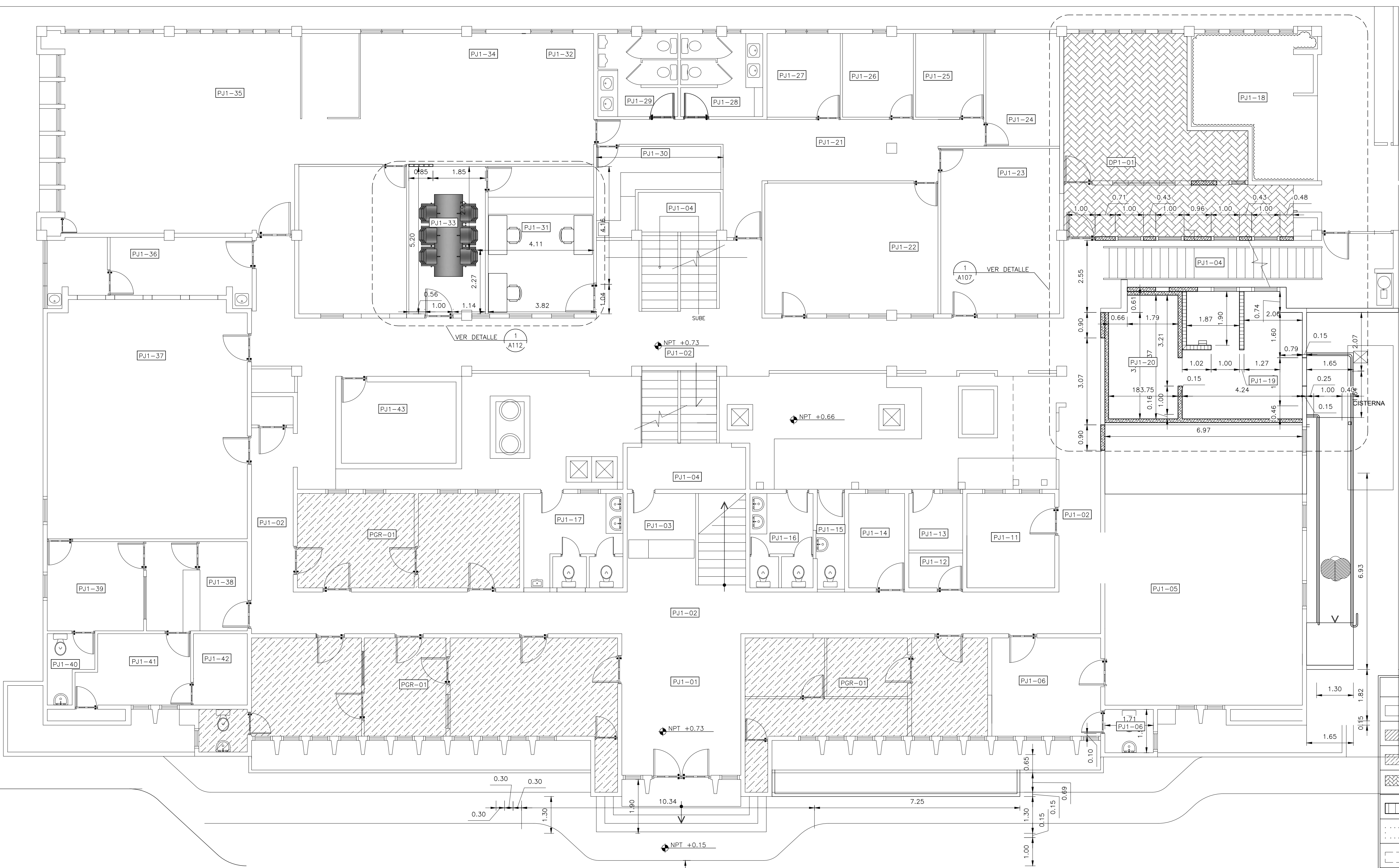
PLANTA DIMENSIONADA PROPUESTA NIVEL 1 ESCALA: 1:75
