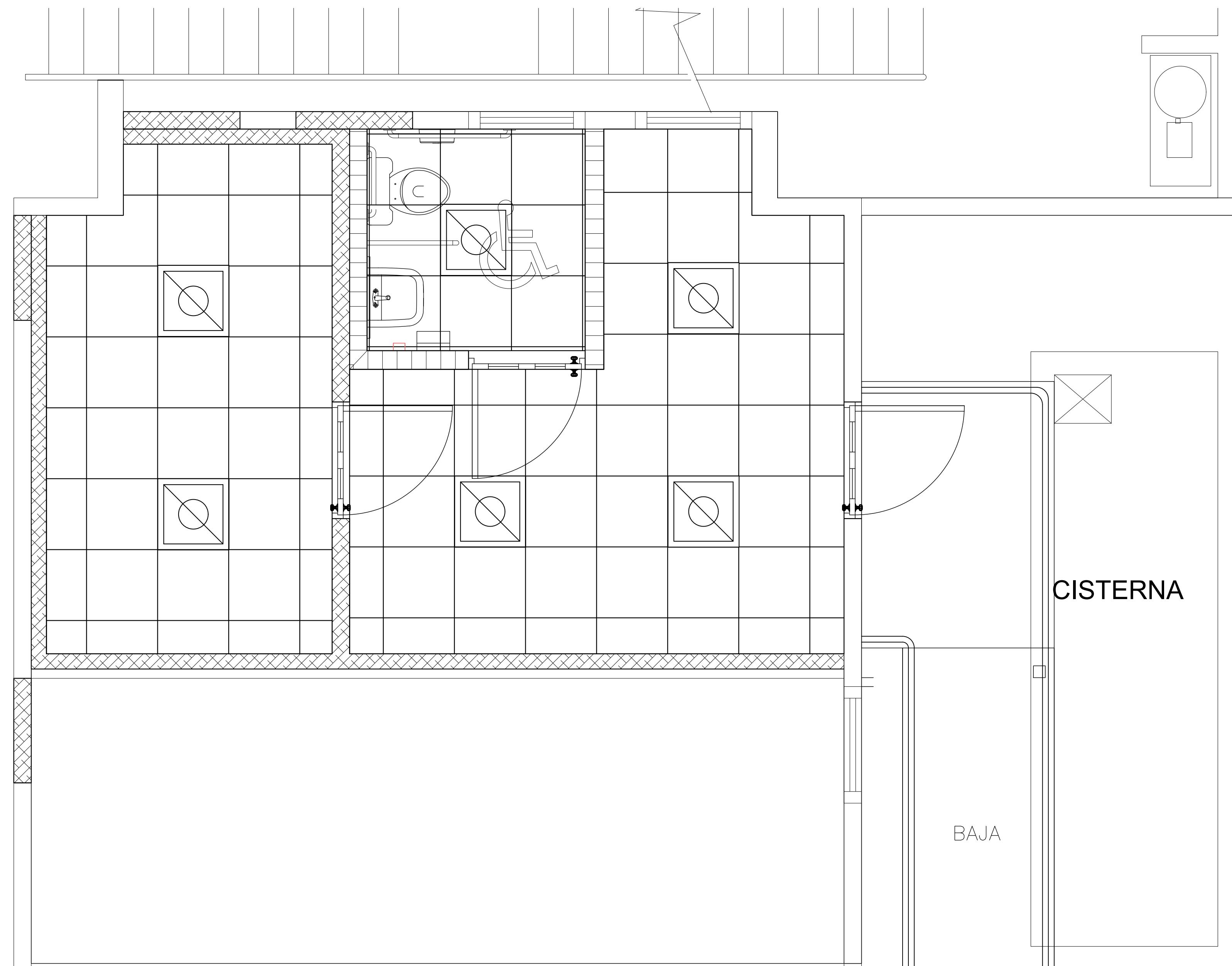
VISTA AMPLIADA PROPUESTA PLANTA DE TECTO SALA DE ENTREVISTAS ESCALA: 1:25
