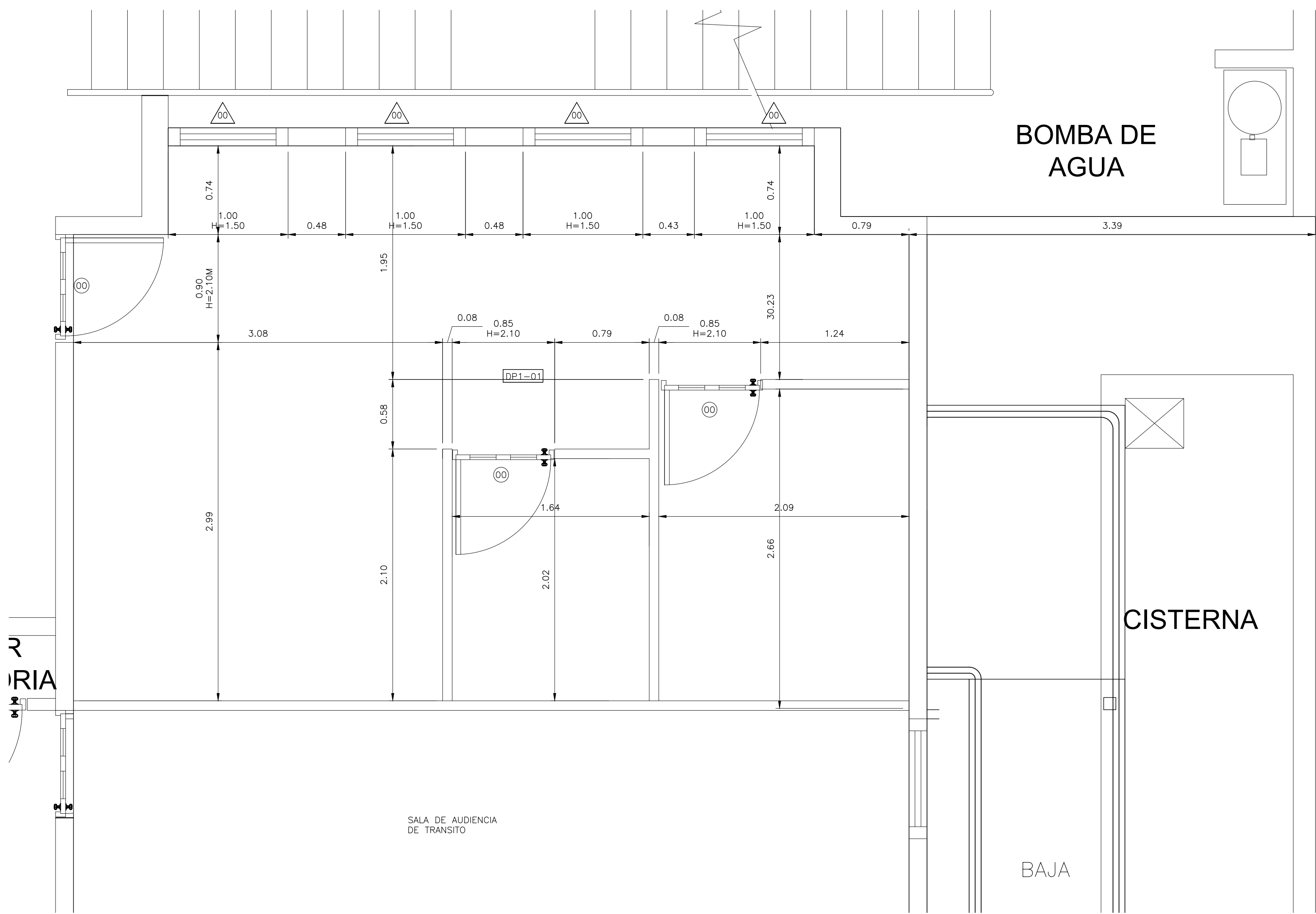
VISTA AMPLIADA AREA DE LA DEFENSA PUBLICA ESCALA: 1:25
