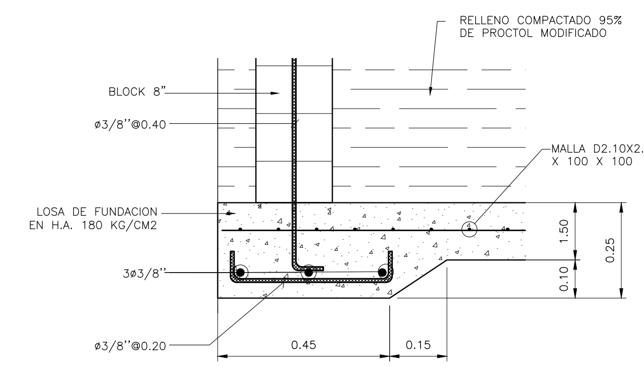
DETALLE DE FUNDACION ESCALA: 1:10
