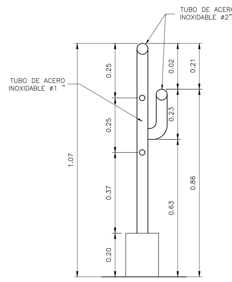
DETALLE BARANDA ESCALA: 1:10
