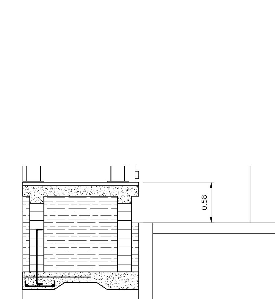
SECCION 1 SALA DE ENTREVISTAS ESCALA: 1:33
