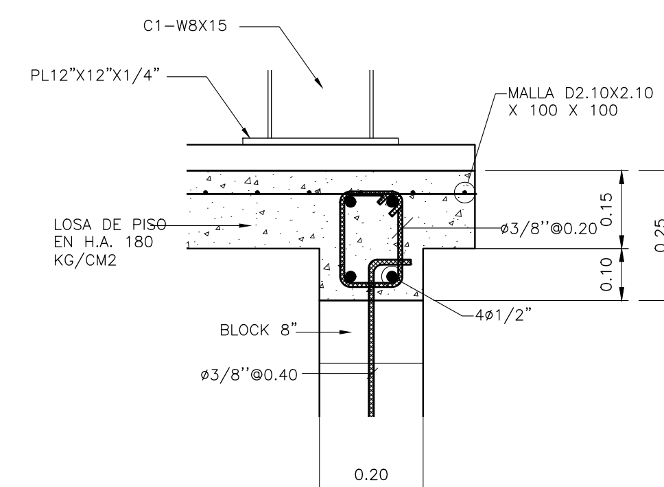
DETALLE DE CONEXION 3 ESCALA: 1:10
