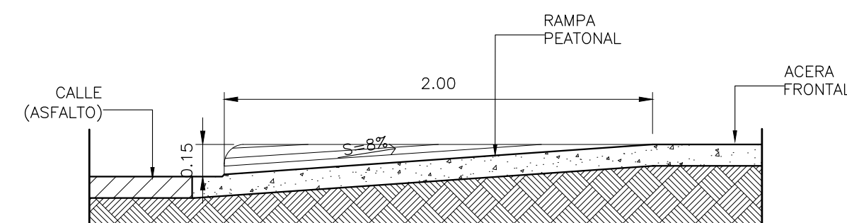
SECCION DE RAMPA PEATONAL DISCAPACITADOS ESCALA: 1:25
