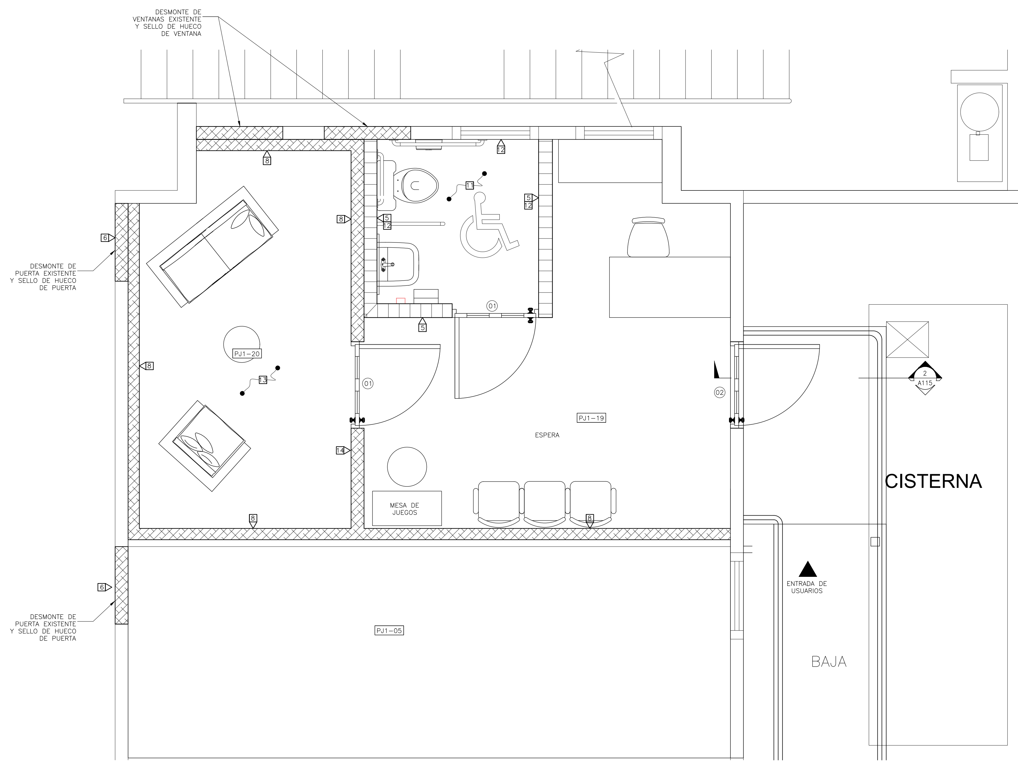
VISTA AMPLIADA PROPUESTA ARQUITECTONICA SALA DE ENTREVISTAS ESCALA: 1:25
