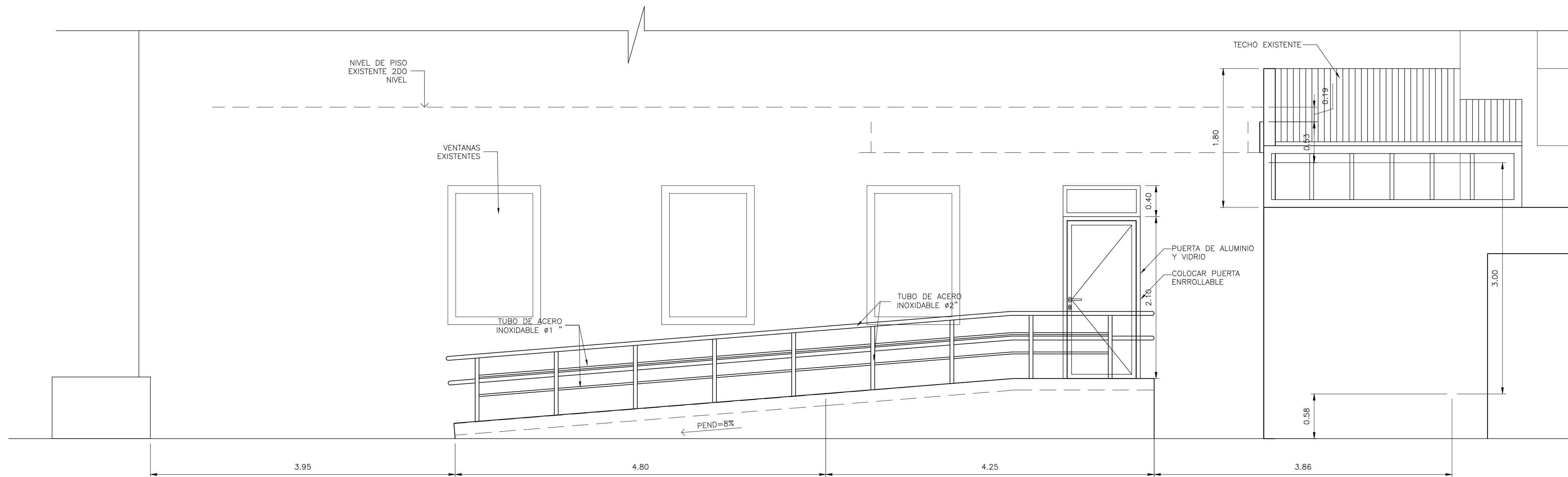
ELEVACION 1 ESCALA: 1:33
