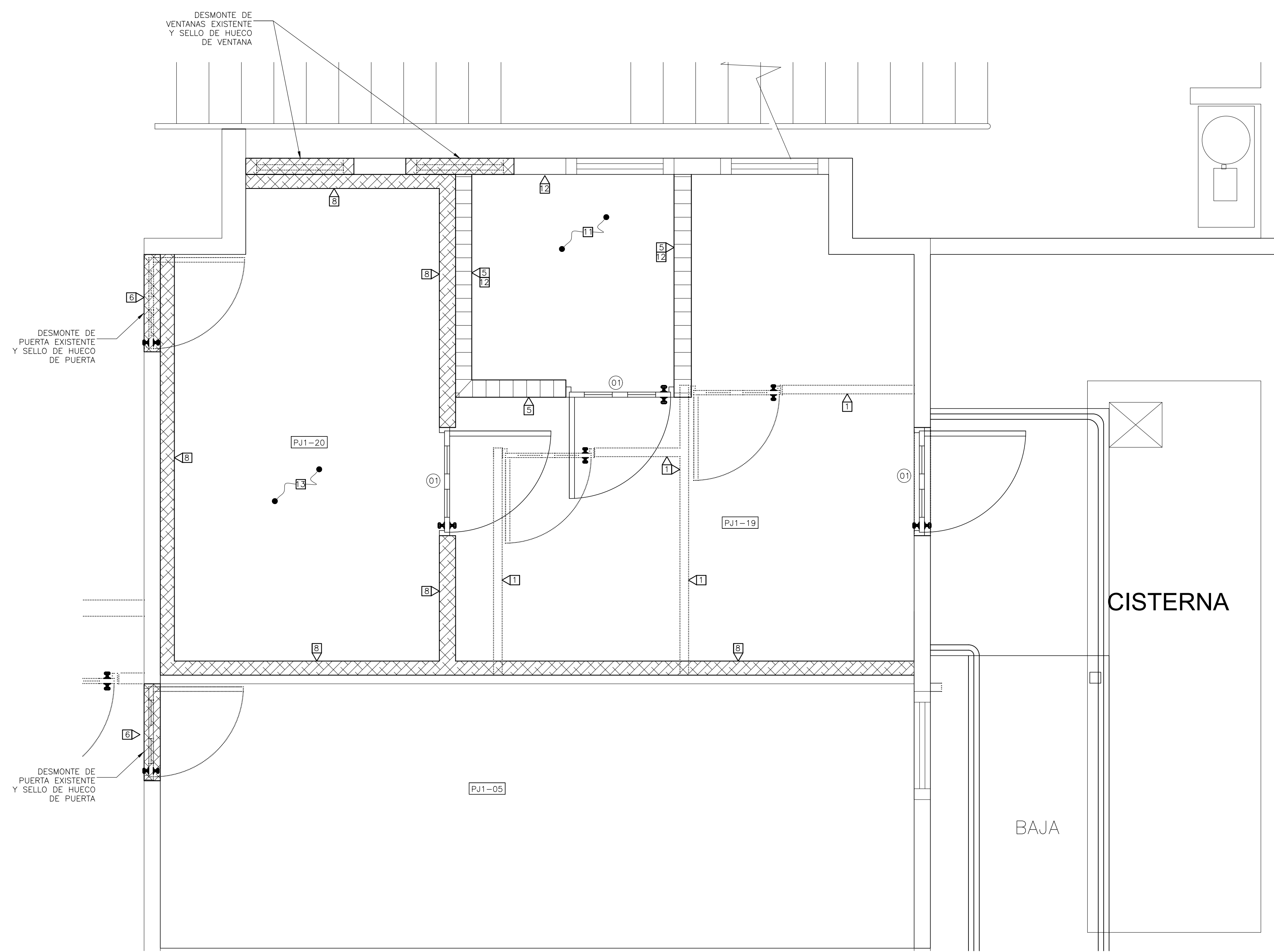
VISTA AMPLIADA AREA DEFENSA PUBLICA PLANTA DE DEMOLICION Y ADICION ESCALA: 1:25
