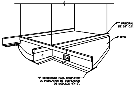
SISTEMA PLAFON SUSPENDIDO 3 ESCALA: NO A ESCALA
