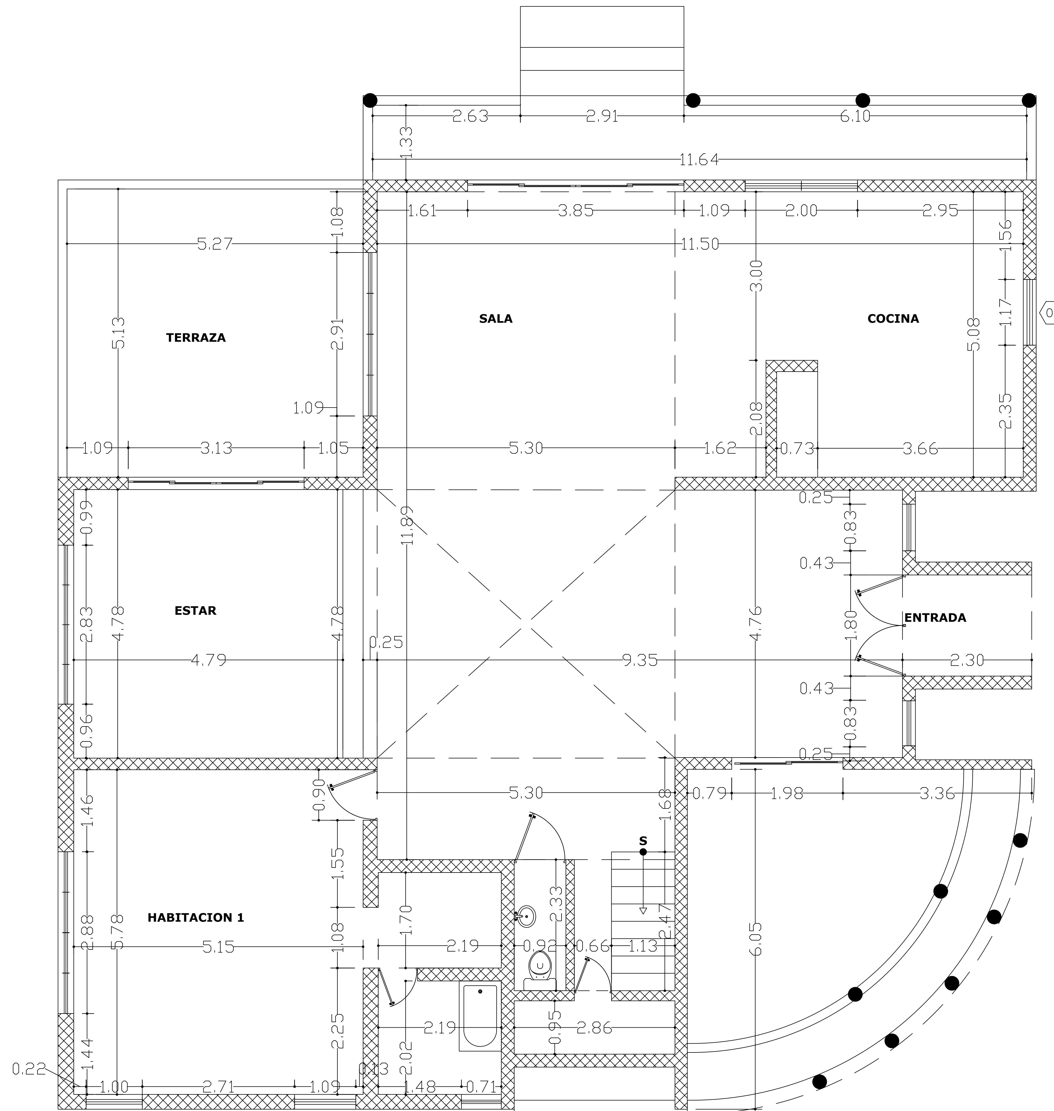
PLANTA DIMENSIONADA ACTUAL N1 ESCALA: 1:1000
