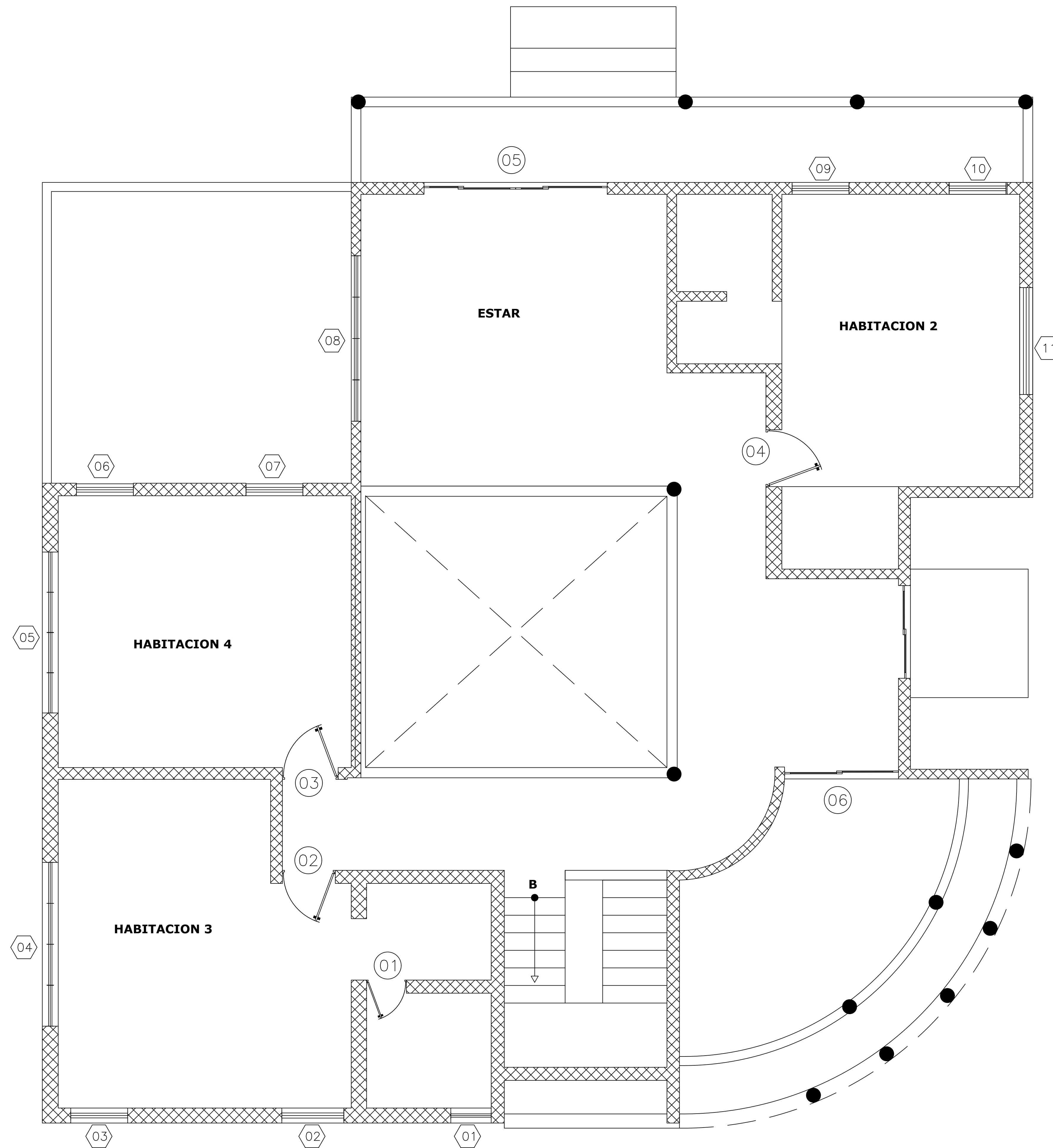
PLANTA ARQUITECTONICA ACTUAL N2 ESCALA: 1:1000
