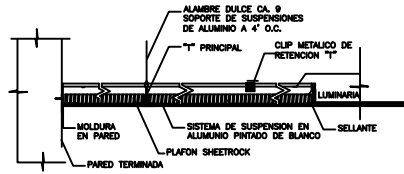
DETALLE INSTALACION PLAFON 6 ESCALA: NO A ESCALA
