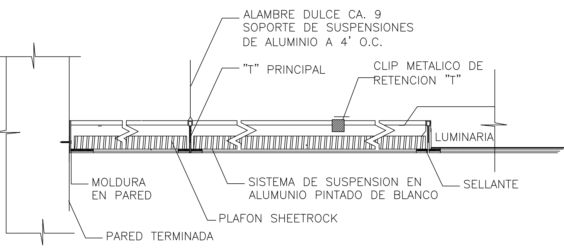
DETALLE DE INSTALACION DE PLAFON ESCALA: 1:50
