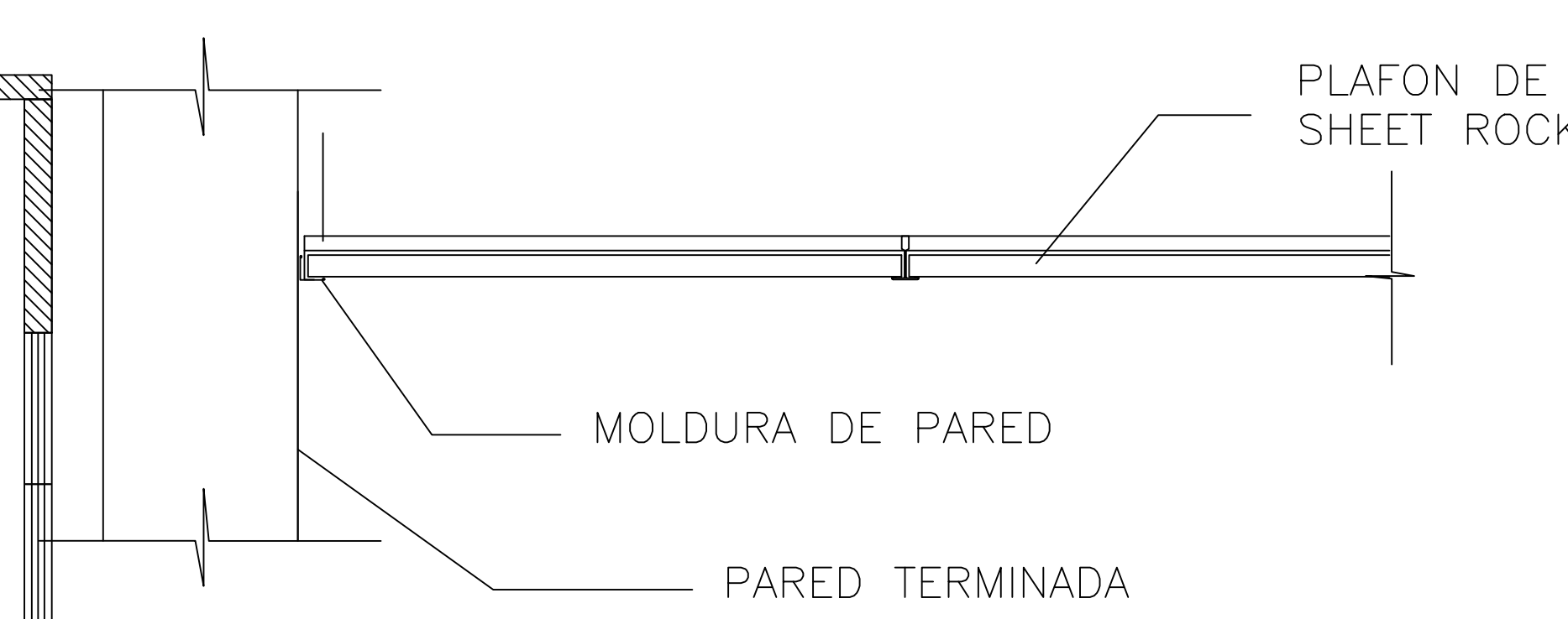
SISTEMA PLAFON SUSPENDIDO ESCALA: 1:50
