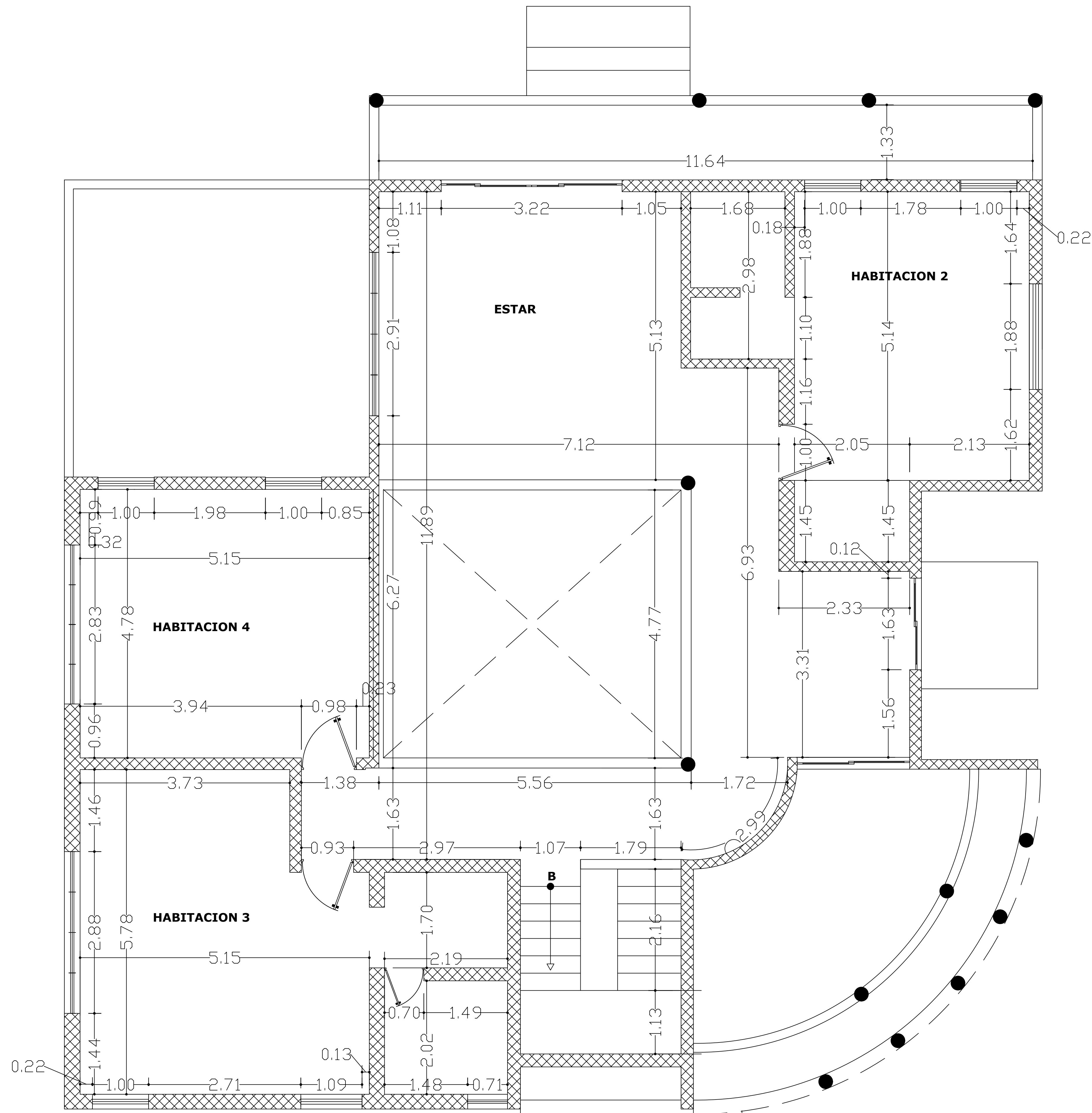
PLANTA DIMENSIONADA ACTUAL N2 ESCALA: 1:1000
