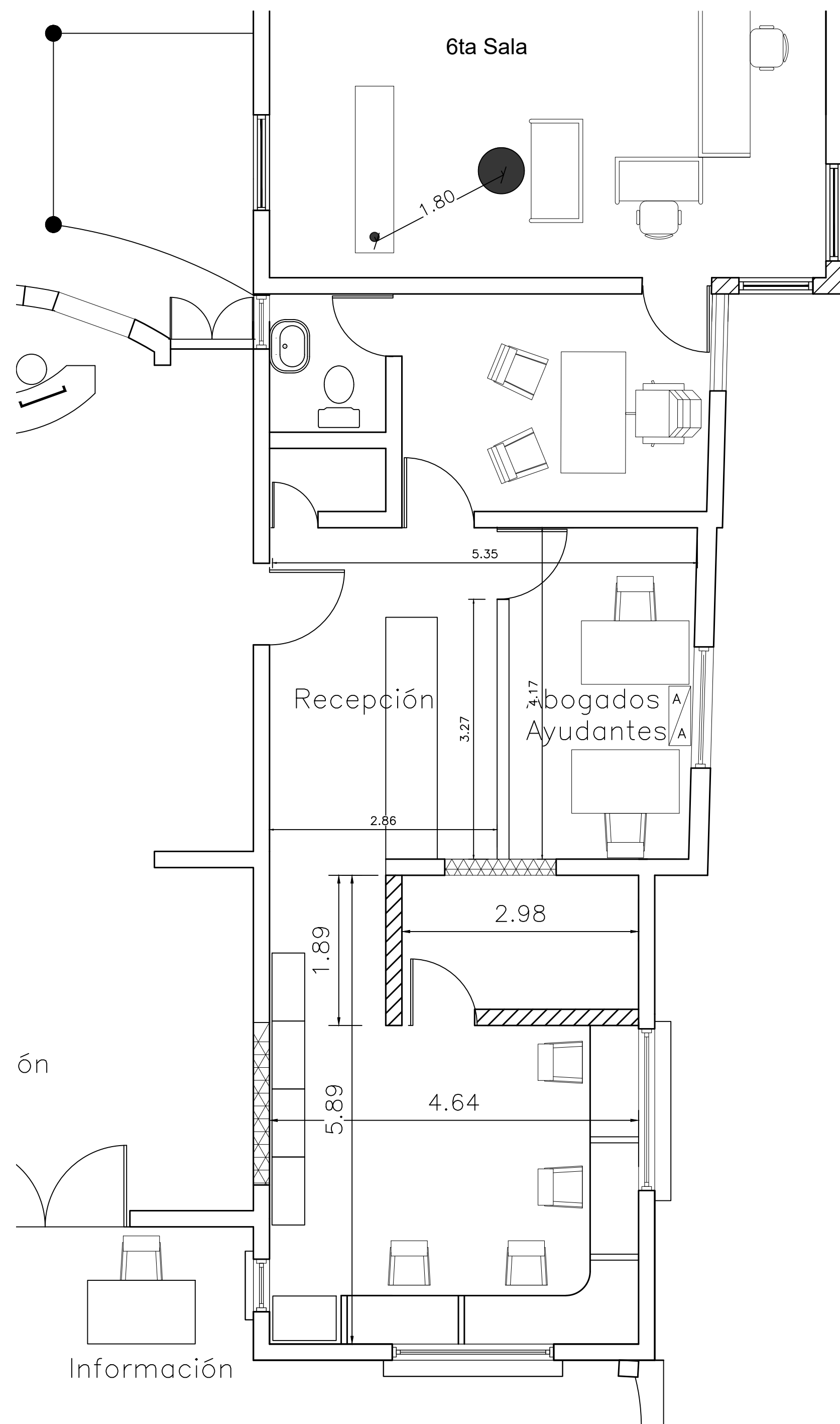
PLANTA ARQUITECTONICA EXISTENTE 6ta Sala ESCALA: 1:100
