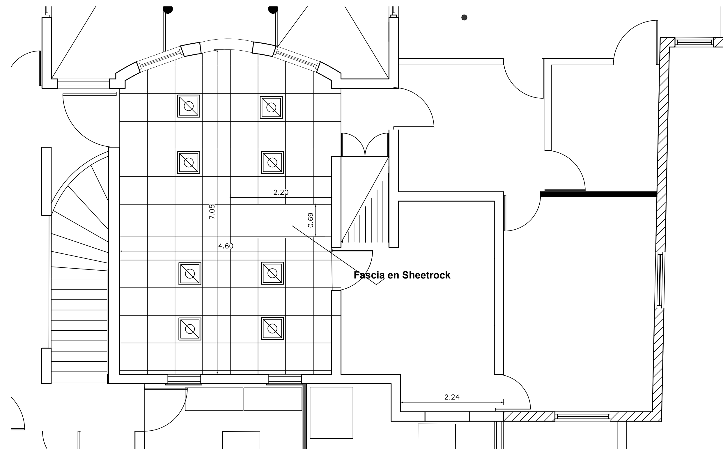
PLANTA DE PLAFOND Y LAMPARAS ESCALA: 1:100
