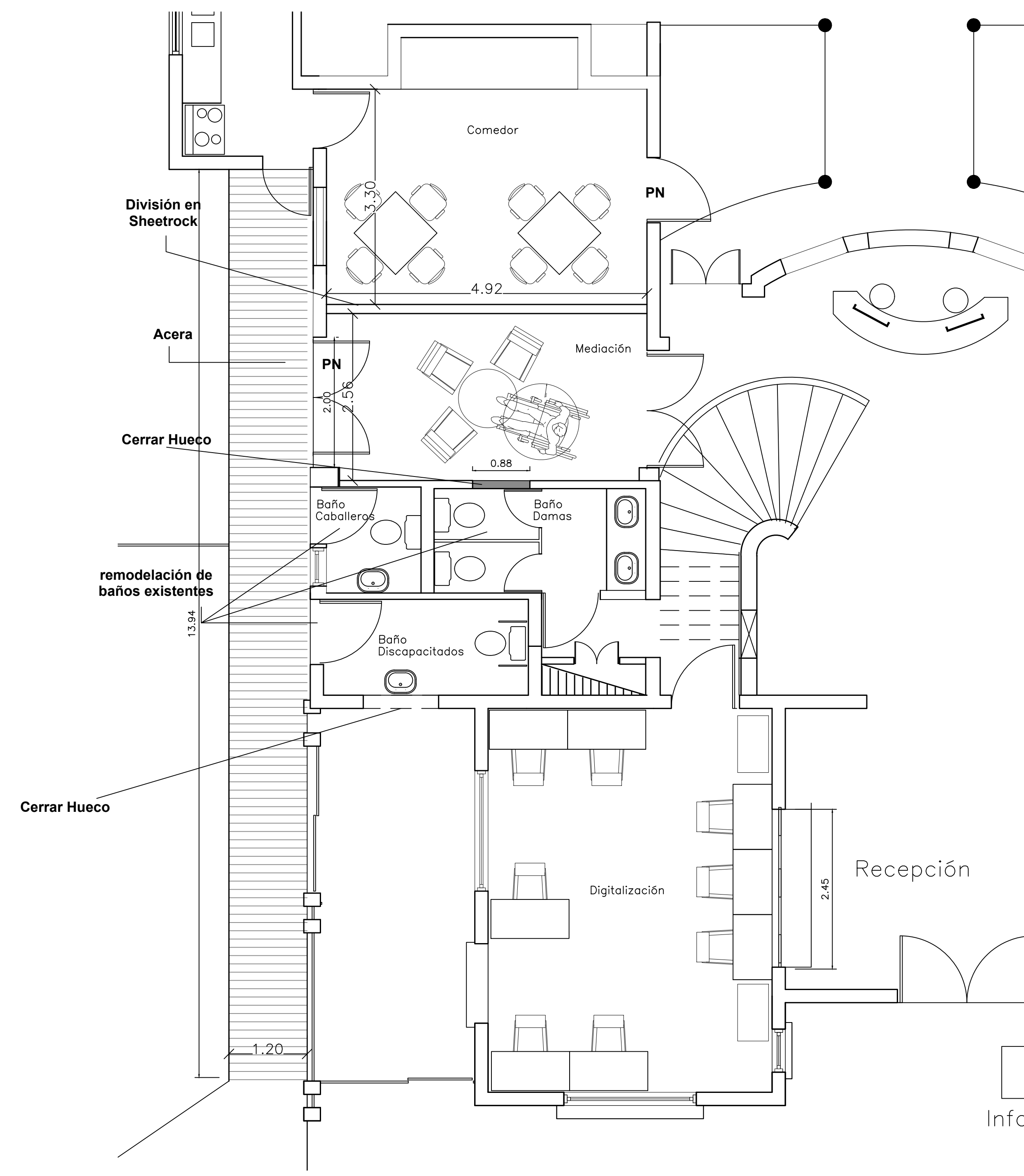
PROPUESTA DE ADECUACION ESCALA: 1:50
