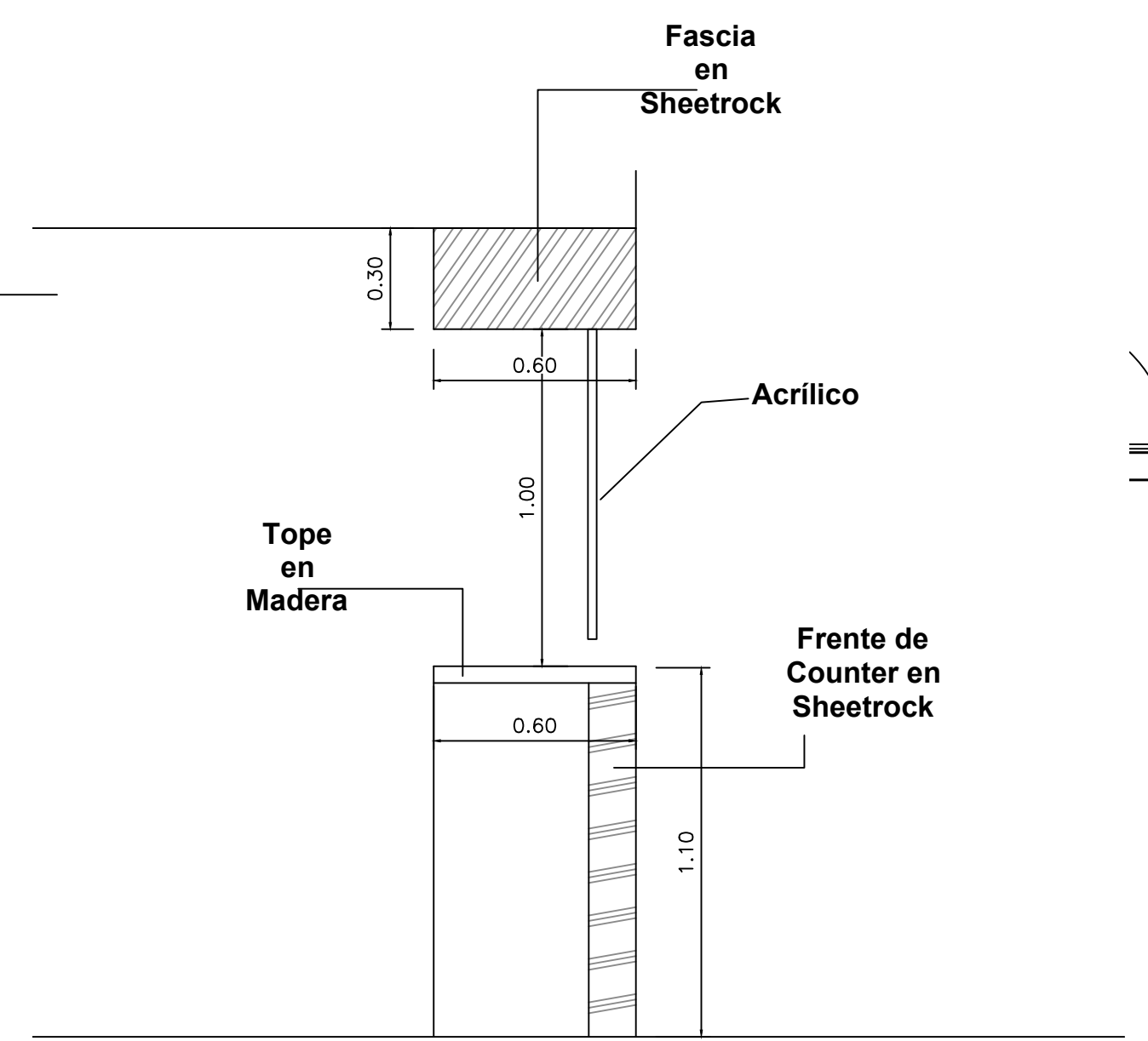
DETALLE DE COUNTER ESCALA: 1:20
