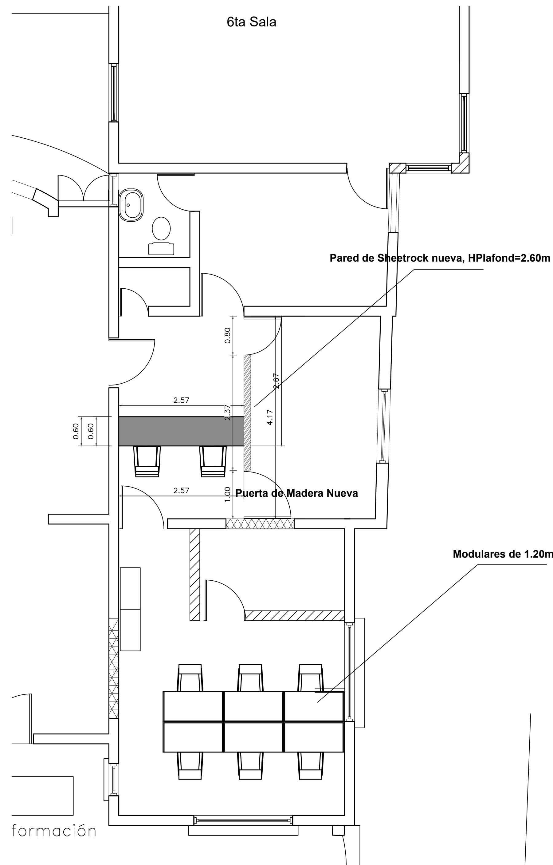
PLANTA ARQUITECTONICA PROPUESTA 6ta Sala ESCALA: 1:100
