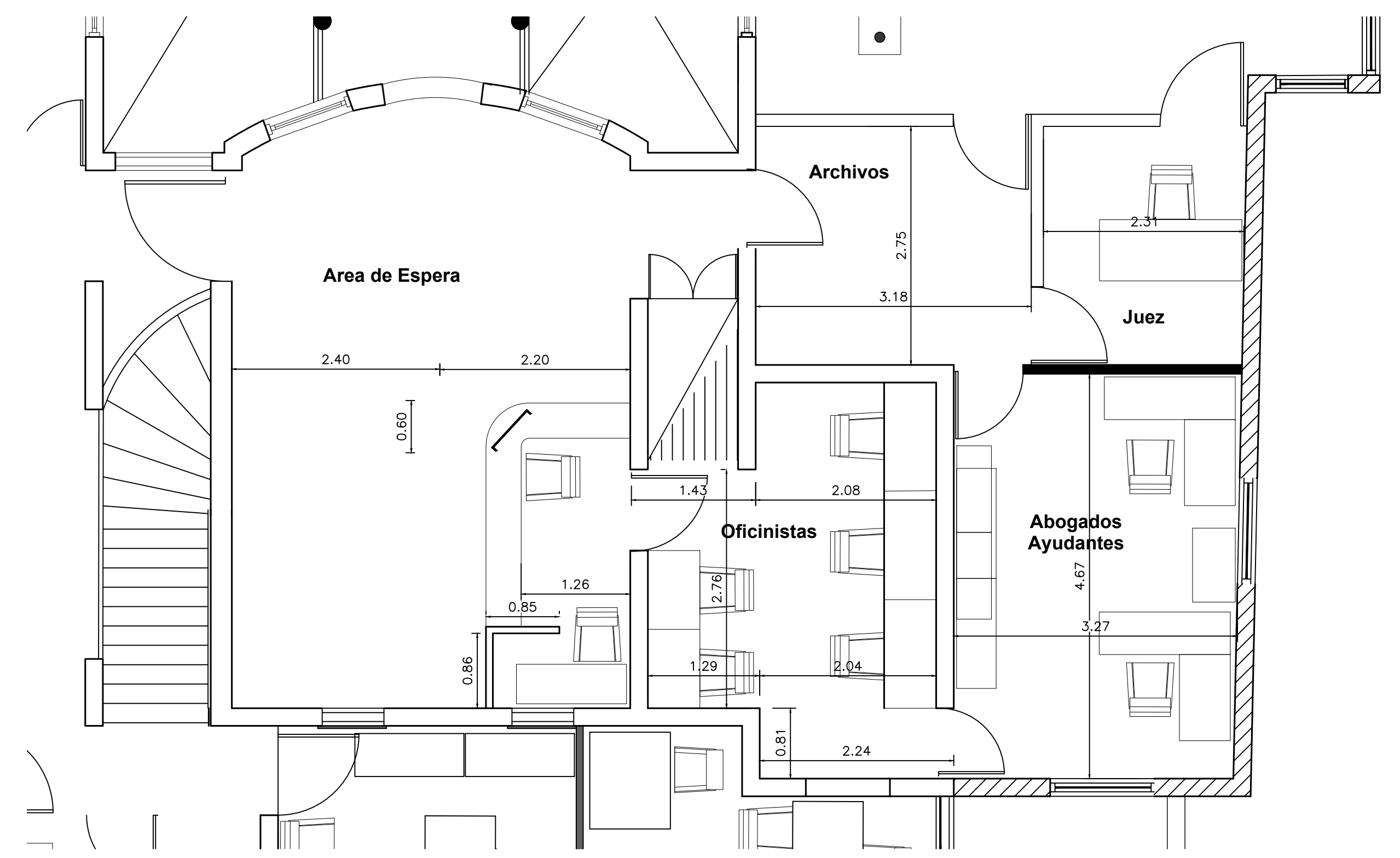
PLANTA ARQUITECTONICA EXISTENTE 8va Sala ESCALA: 1:100
