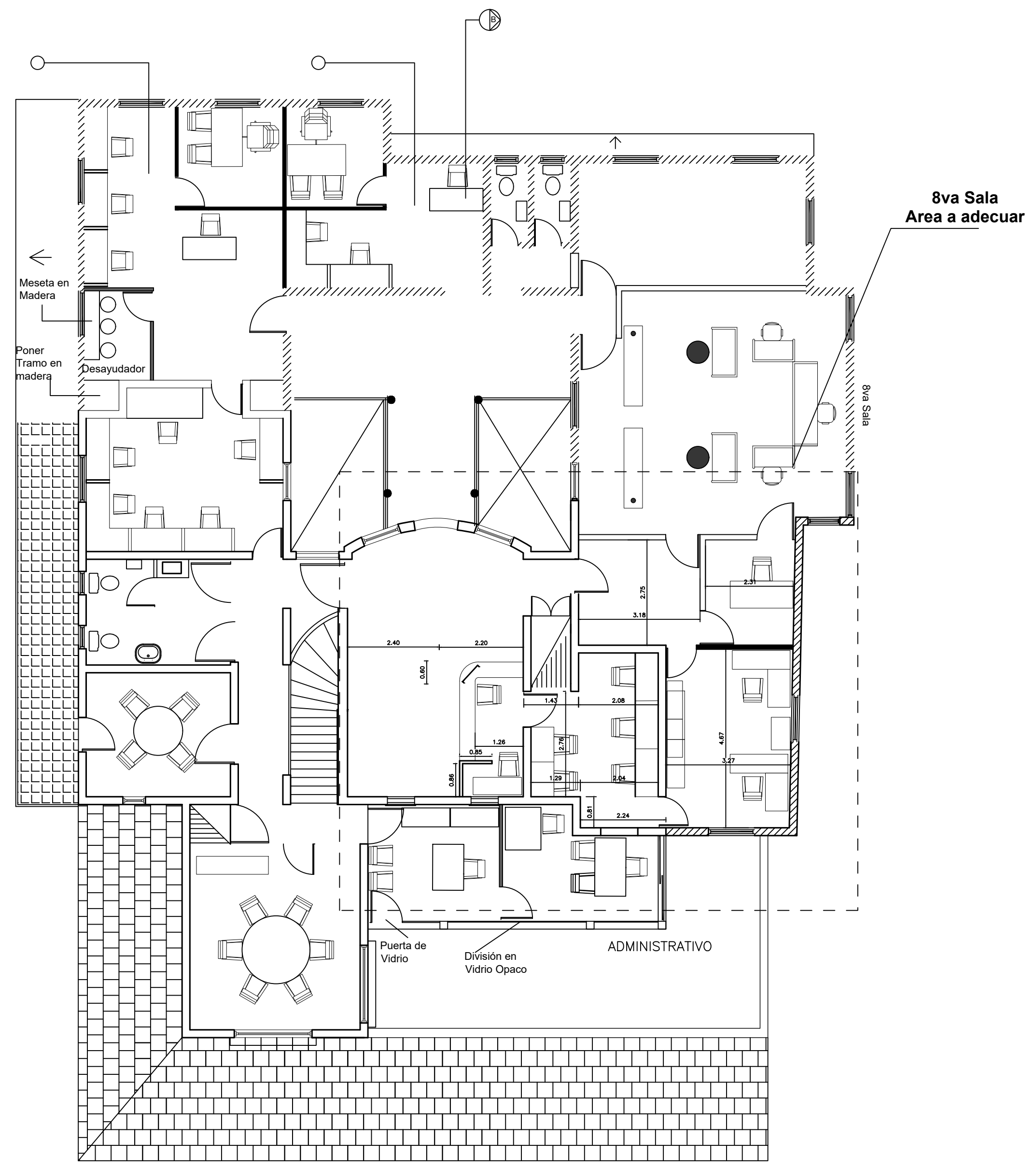
PLANTA ARQUITECTONICA SEGUNDO NIVEL
