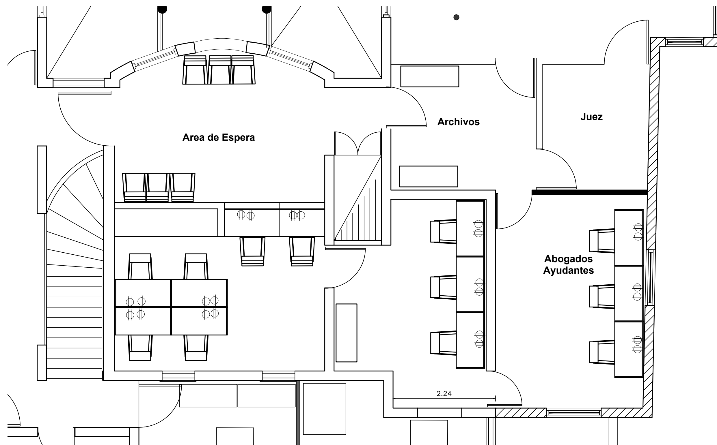
PLANTA ELECTRICA ESCALA: 1:100
