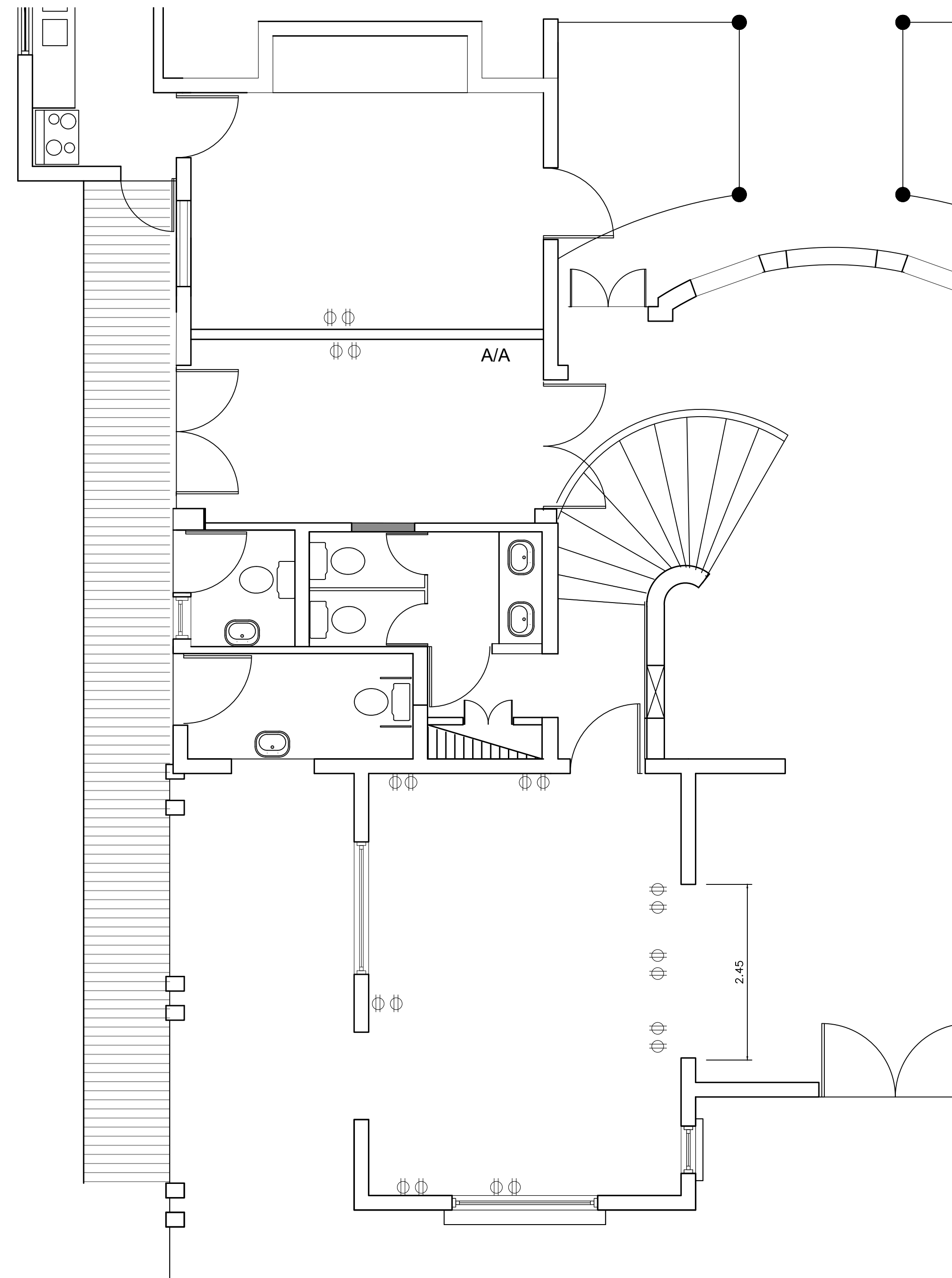
PLANTA ELECTRICA ESCALA: 1:50
