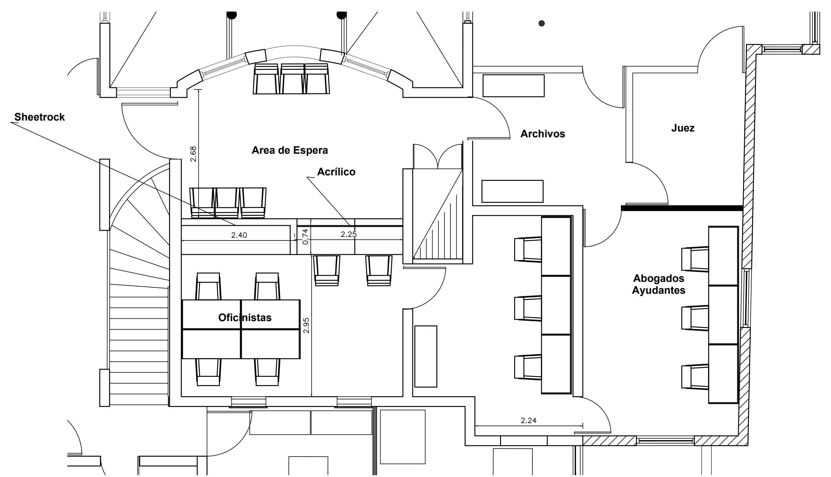
PLANTA ARQUITECTONICA PROPUESTA 8va Sala ESCALA: 1:100
